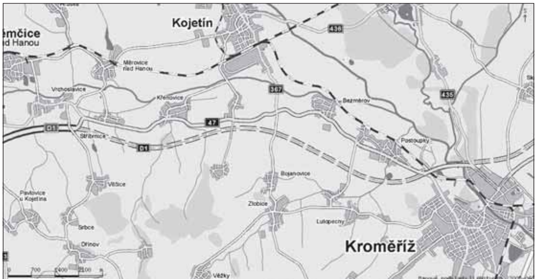
Plánovaná trasa dálnice D1 v úseku Kojetín - Kroměříž západ.
