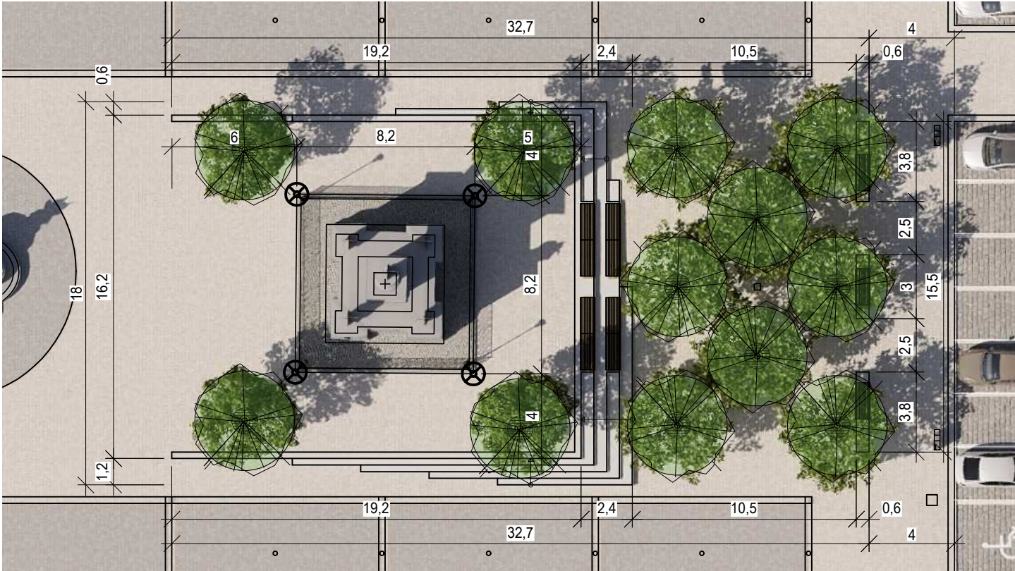
PŮDORYS STŘEDOVÉ ČÁSTI NÁMĚSTÍ
