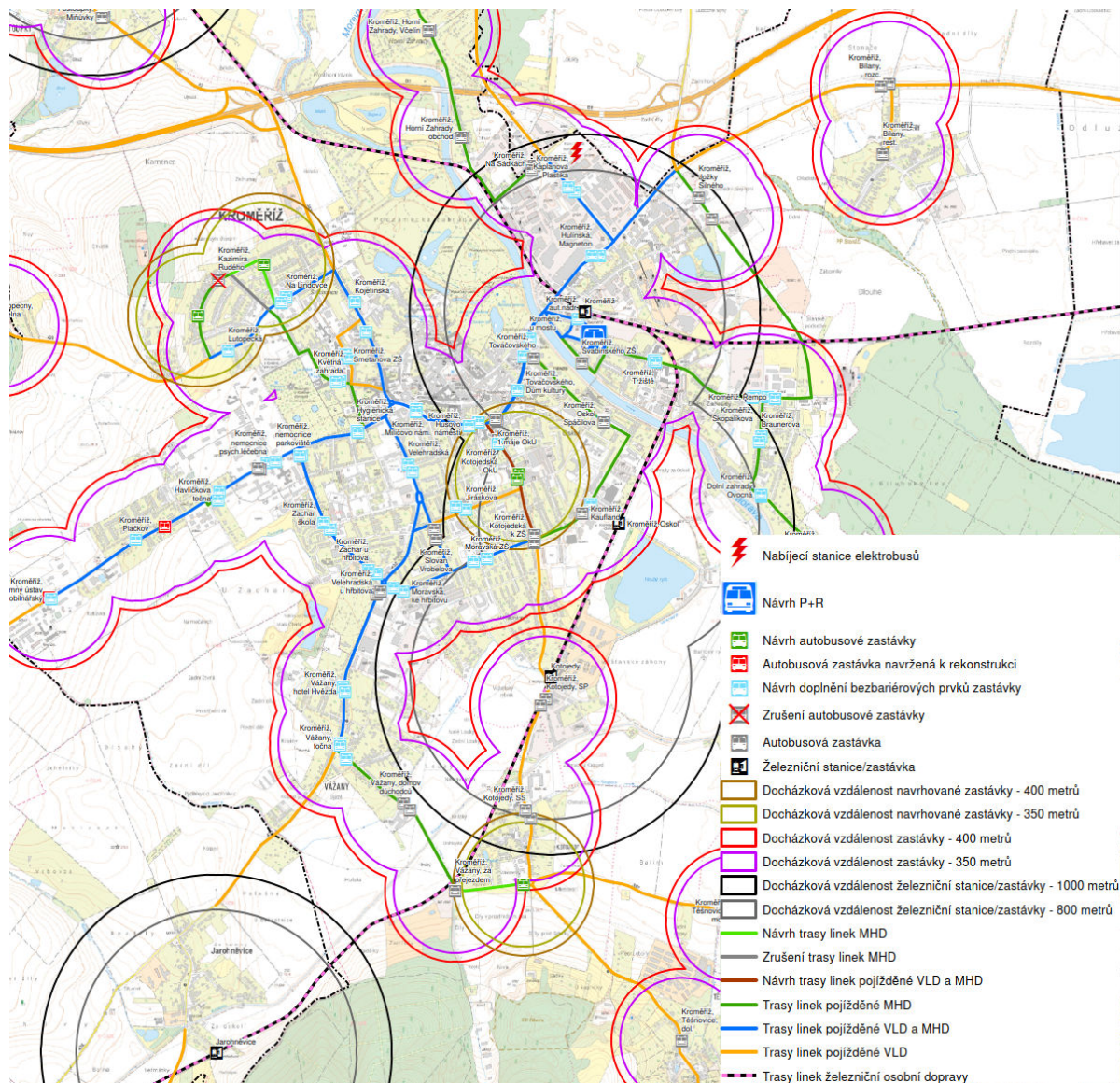
Obrázek 5 Návrh úpravy koncepce veřejné dopravy
